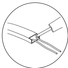
Saldare il connettore sulle piazzole
